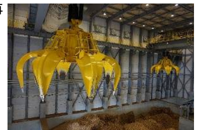
木材チップを貯蔵する燃料倉庫
