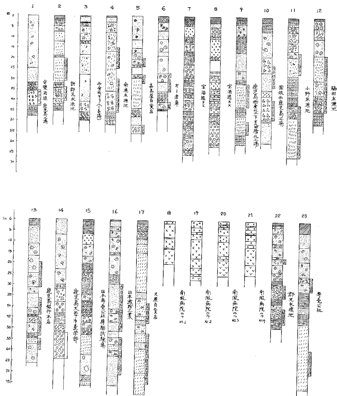
鹿児島市中内ホーリング地質柱状図
