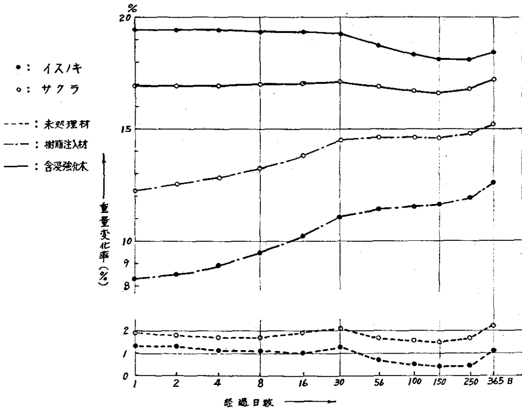
図2. イスノキ, サクラ材の経時的重量の変化率
