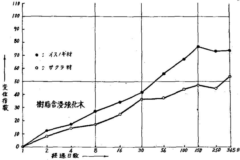
図1. イスノキ, サクラ樹脂含浸強化木の経時的変位指数の変動
