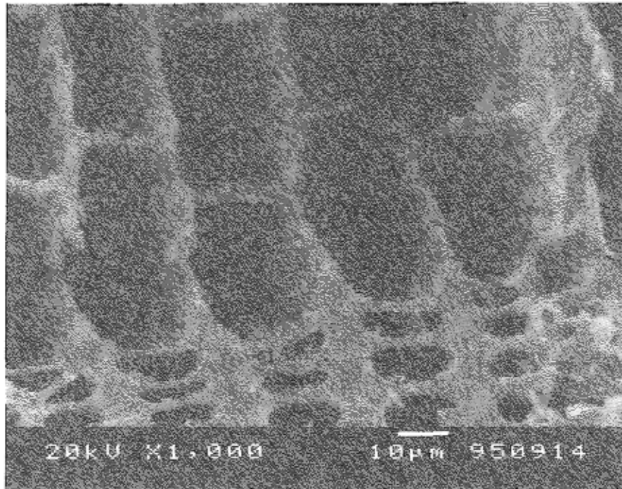
黒炭（クロマツ）のSEM写真
