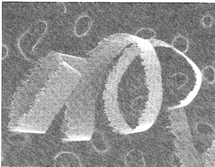
単結晶ダイヤモンド平バイトによる超精密切削加工の切りくず (AI)
