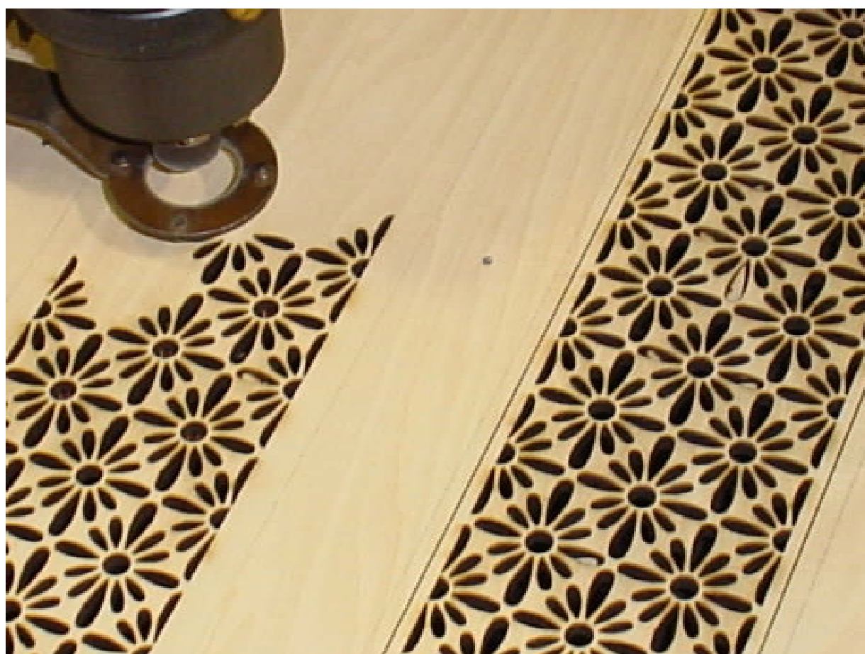
炭酸ガスレーザーによる仏壇彫刻部品の加工
