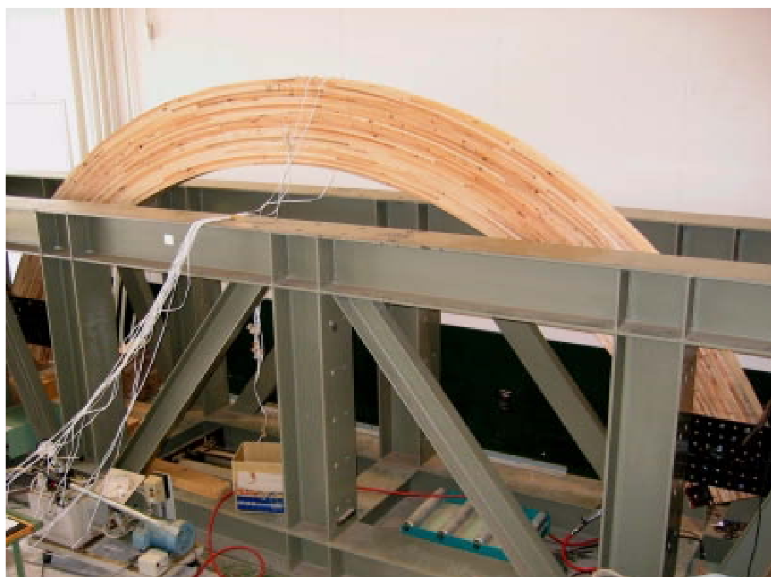
スギ湾曲集成材の強度試験
