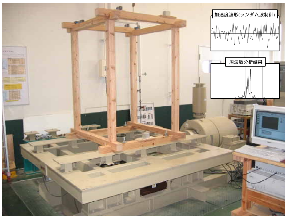
立体フレームの振動試験
