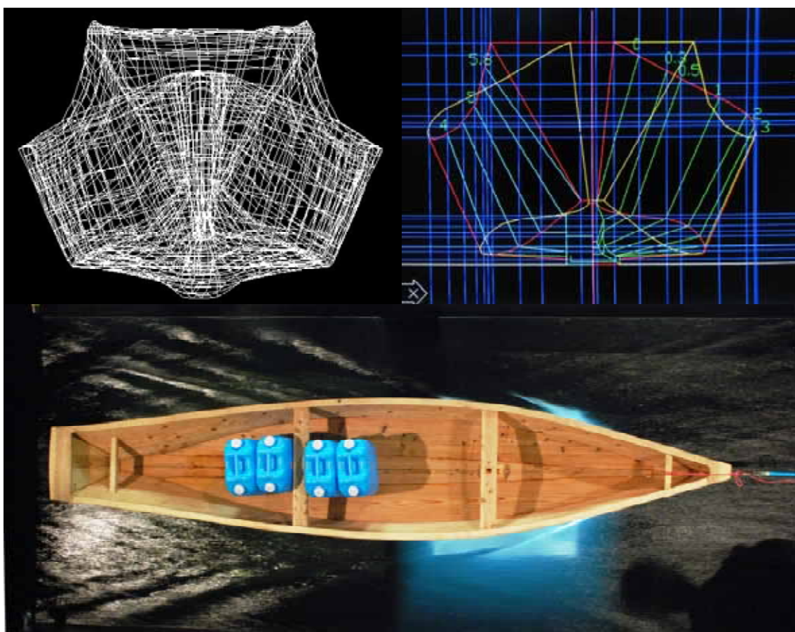
伝統木造船の小型版“クッカル”の開発
