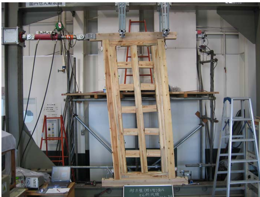
格子パネルにより補強した耐力壁の面内せん断試験
